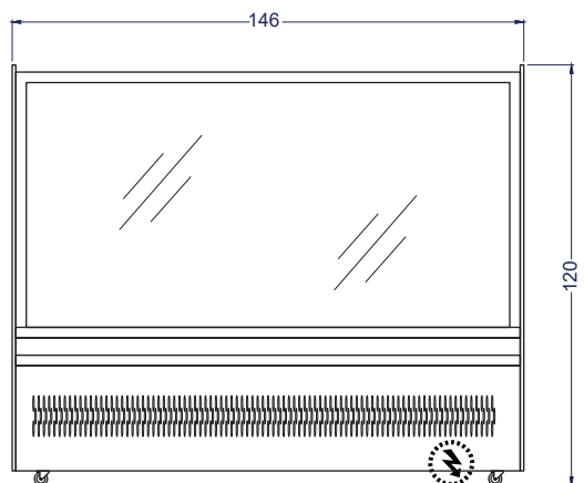
Vista Elevación
