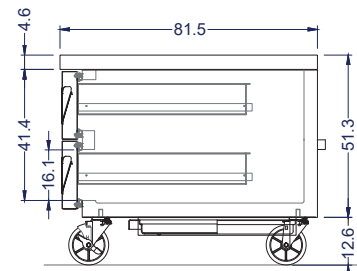
Vista Derecha
