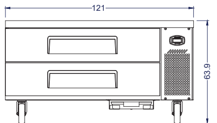
Vista Elevación
