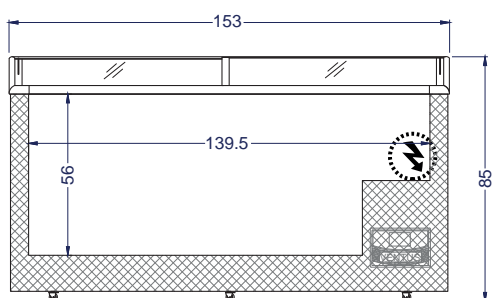
Vista Elevación
