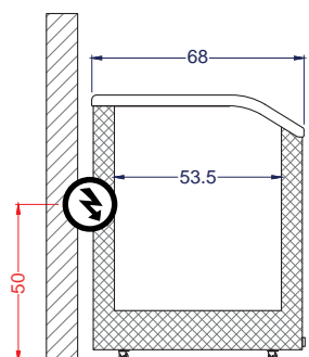
Vista Izquierda
