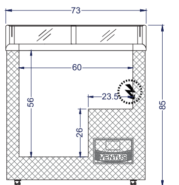
Vista Elevación
