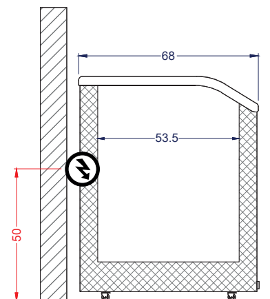
Vista Izquierda
