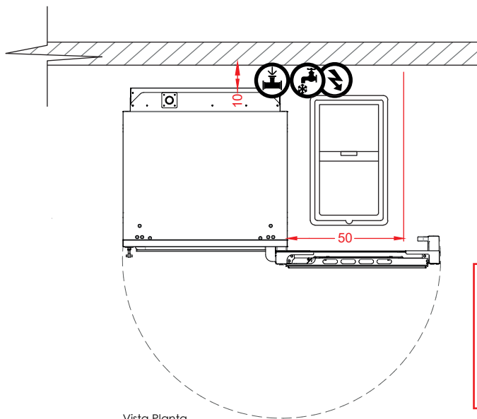
Vista Planta
