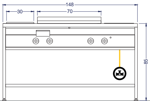
Vista Elevación
