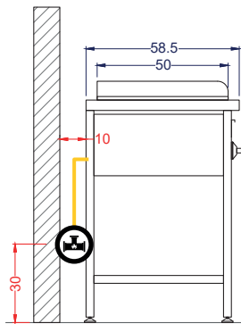
Vista Izquierda
