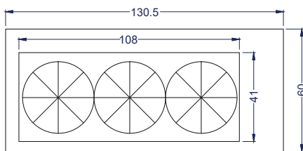
Vista Planta Medidas internas
