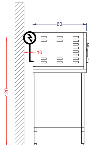
Vista Izquierda
