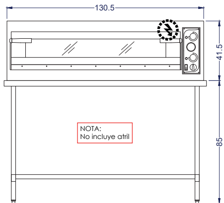
Vista Elevación
