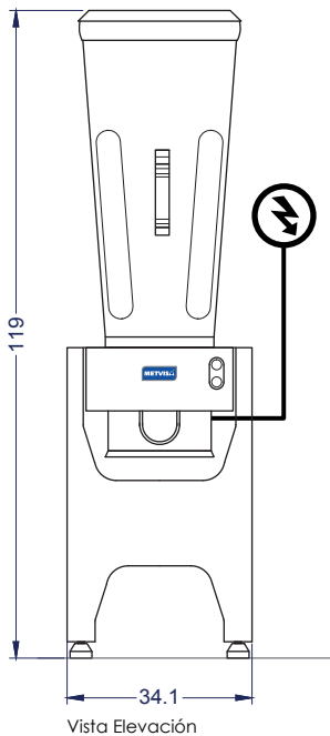
Vista Elevación
