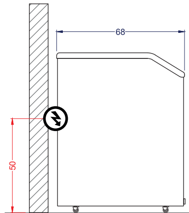
Vista Izquierda
