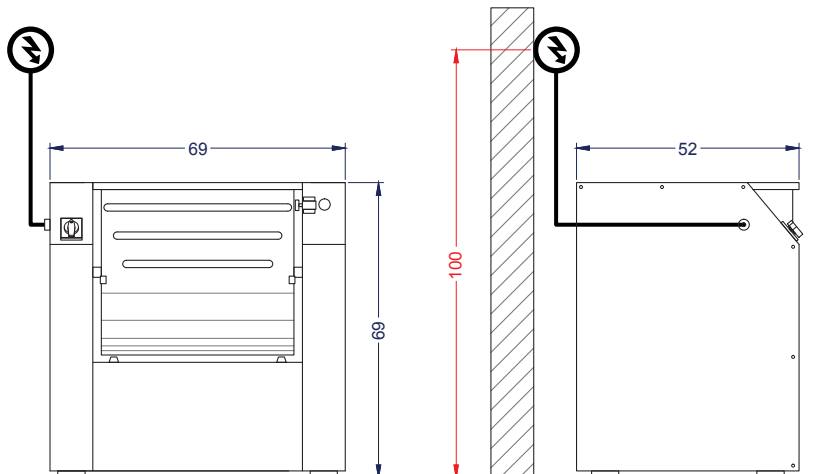
Vista Elevación
