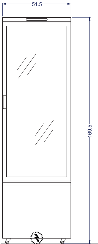
Vista Elevación
