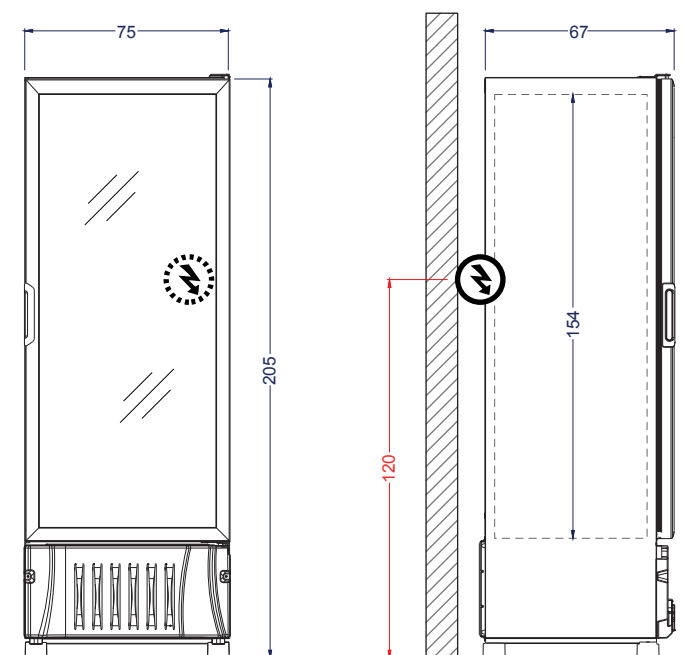
Vista Elevación
