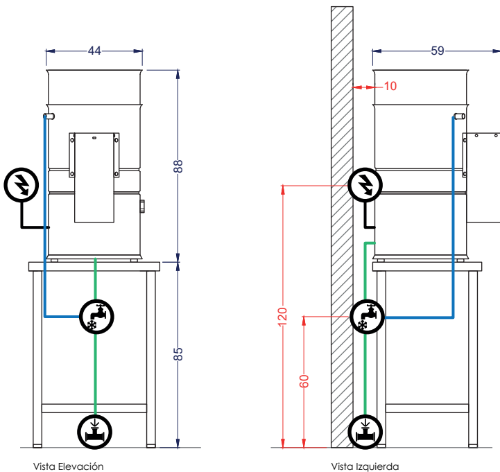
Vista Elevación
