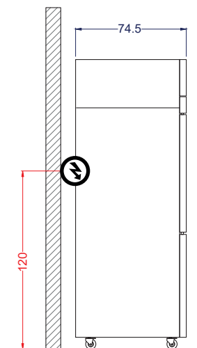
Vista Izquierda
