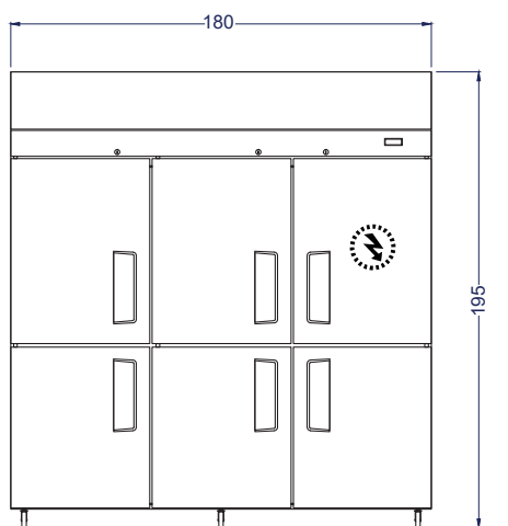
Vista Elevación
