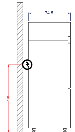
Vista Izquierda
