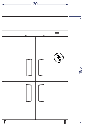
Vista Elevación
