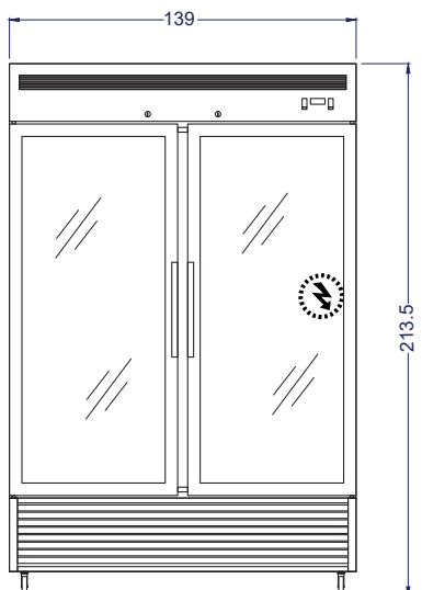
Vista Elevación
