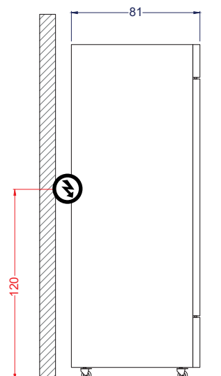
Vista Izquierda
