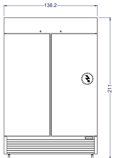
Vista Elevación
