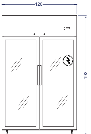
Vista Elevación
