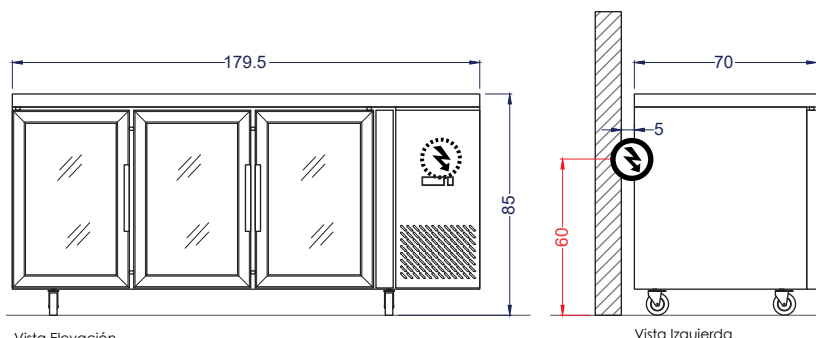
Vista Elevación
