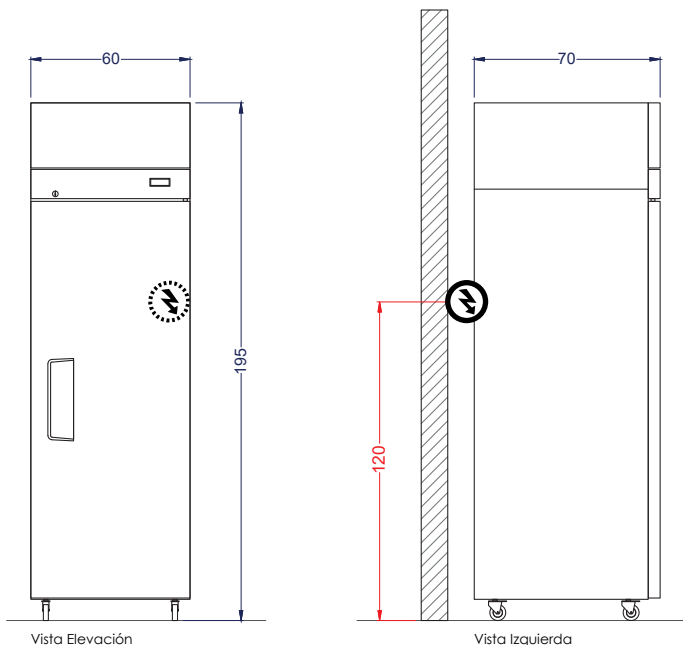
Vista Elevación
