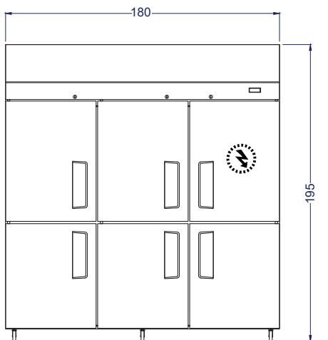
Vista Elevación
