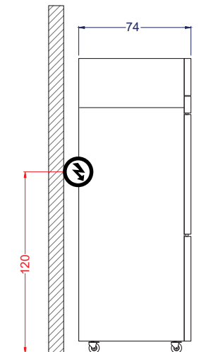
Vista Izquierda
