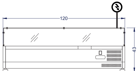
Vista Elevación
