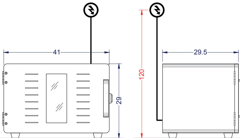
Vista Elevación
