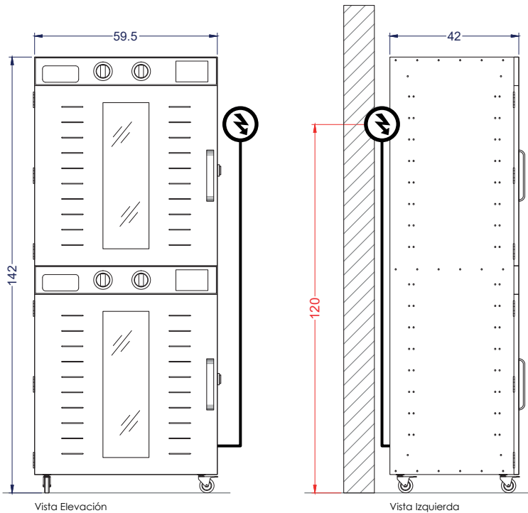
Vista Elevación
